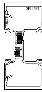
4 SF1878T / SF1857T
