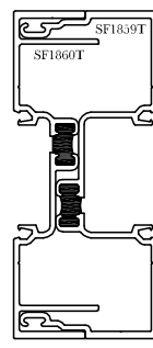
3 SF1859T / SF1860T
