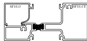
6 SF1851T / SF1853
