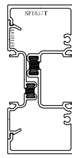
2 SF1857T / SF1854T
