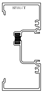
1 SF1857T
